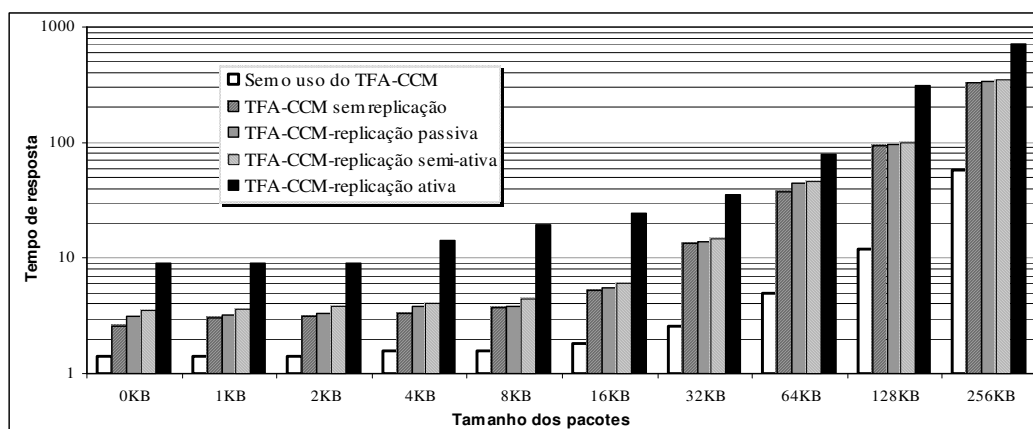
Figura 7. Desempenho do TFA-CCM com diferentes técnicas de replicação
