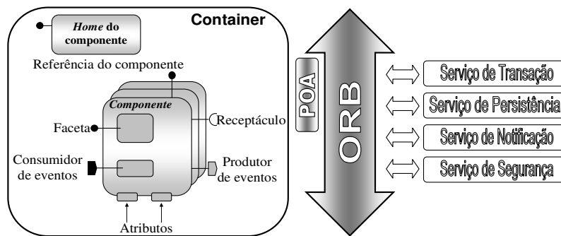
Figura 1. Modelo de Componentes CORBA
