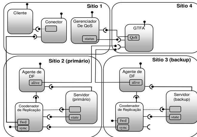
Figura 2. Visão geral do TFA-CCM
