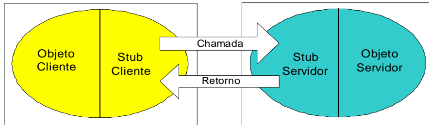
Figura 10.12 – Java/RMI.
